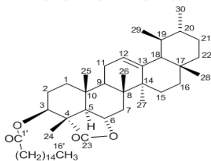
3-Palmityl- \alpha -amyrin-23,6 \alpha -olide (3)
